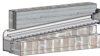
Drainstukje t.b.v. Kopschot model1
